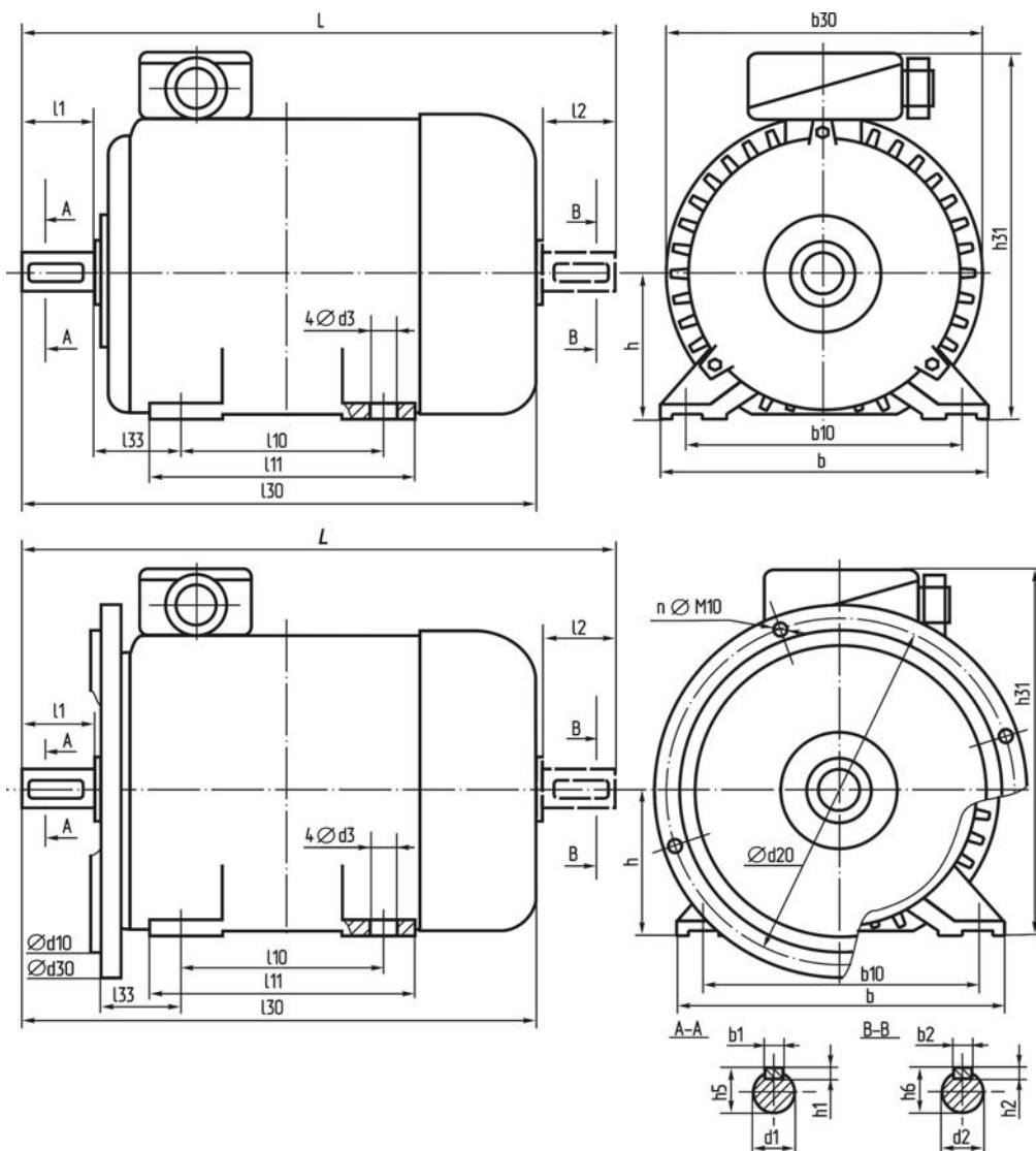
Габаритные, установочные и присоединительные размеры. Электродвигатели малой мощности. IM 1081, IM 1082, IM 2081, IM 2082.
